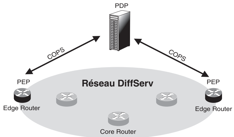
Figure Q.47 Architecture COPS-PR pour un réseau DiffServ
