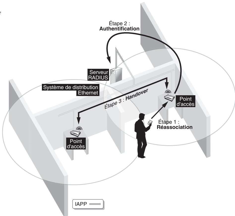
Figure O.10 Le mécanisme de handover d'IAPP
