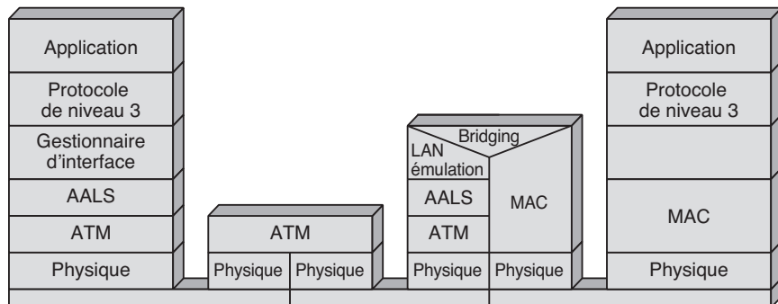
Figure I.4 Architecture de l'émulation de réseaux locaux LANE
